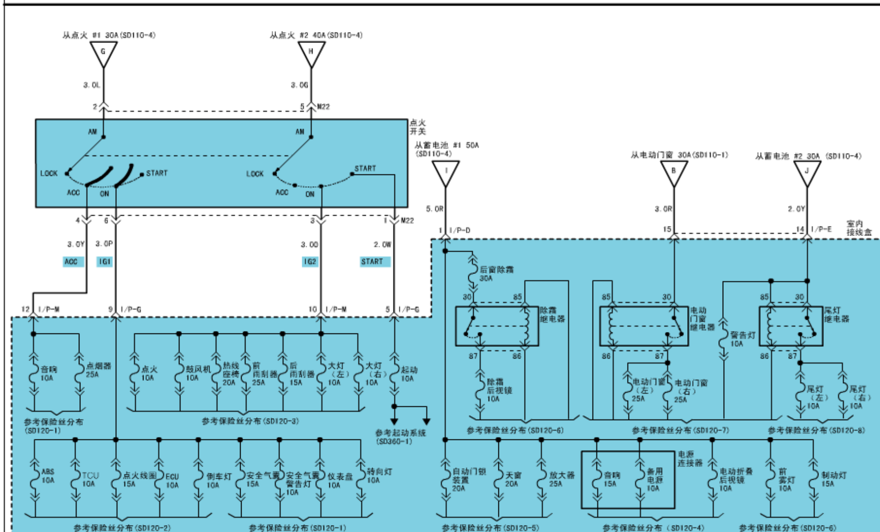
电源分布 (5)
