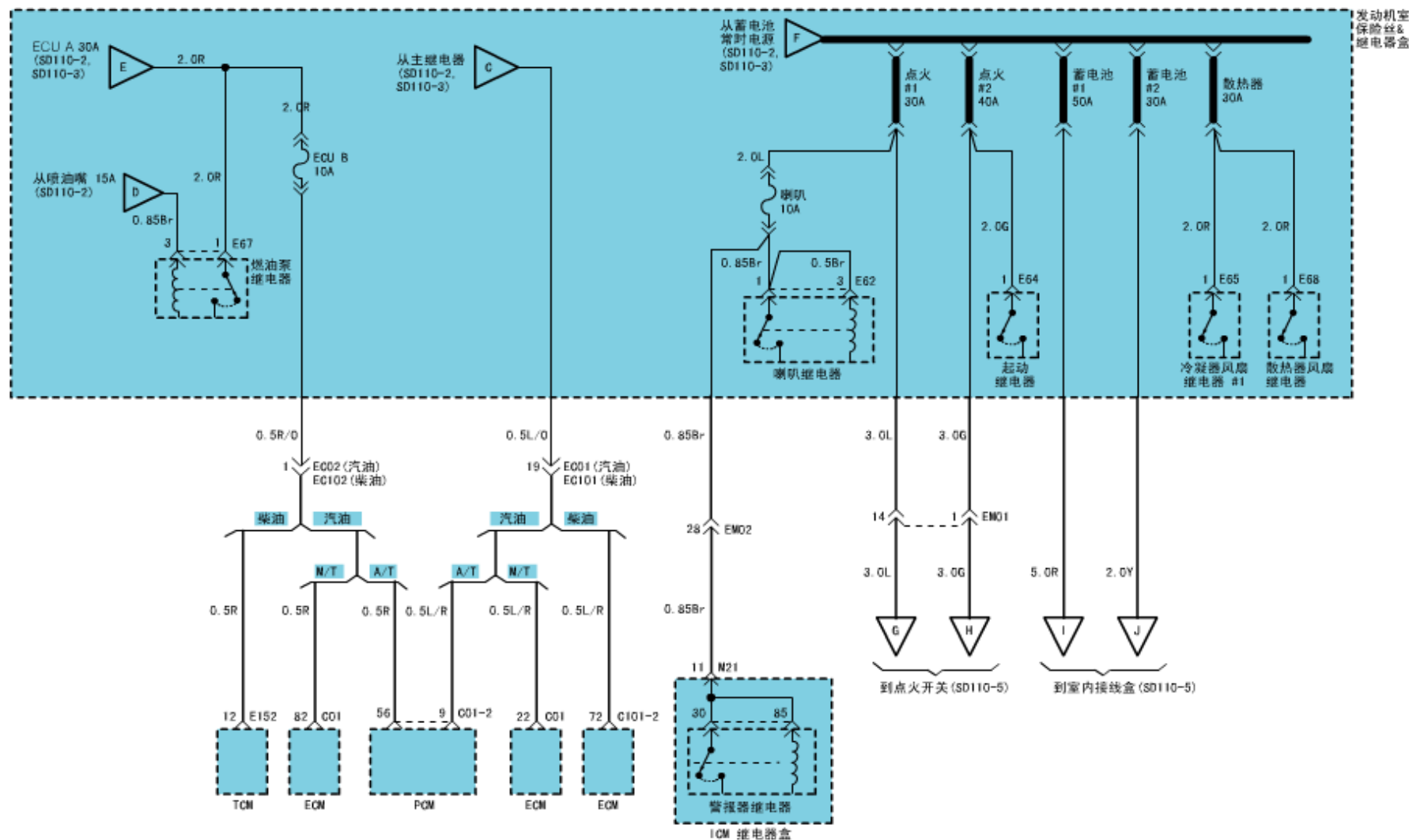
电源分布 (4)
